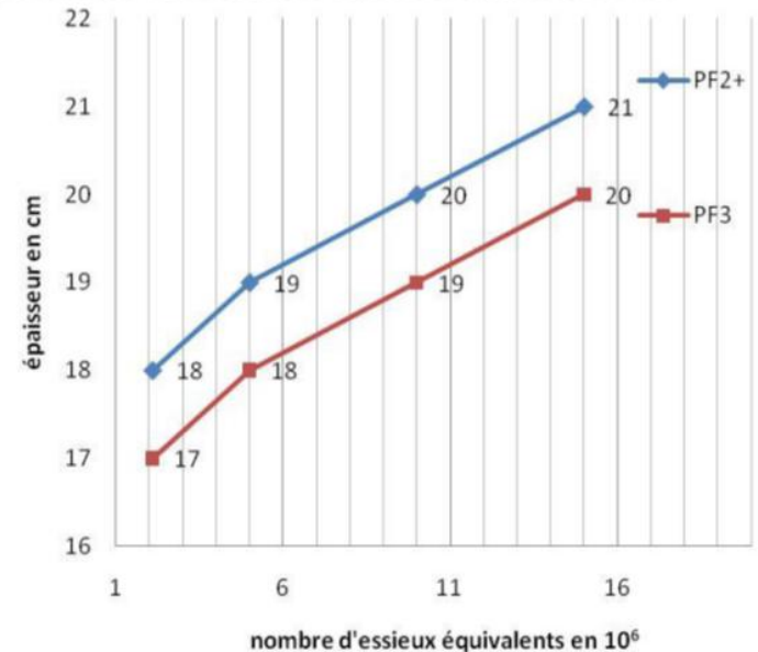
BC5 goudonné sur 10 cm GB3, épaisseur de béton en fonction de NE
