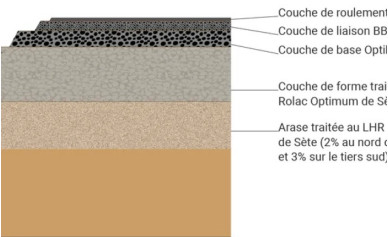
Coupe en travers-type de la chaussée.
