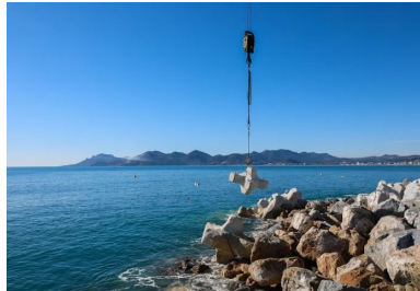
Numéroté et pesé, chaque bloc est placé sur la digue selon un plan de calepinage très précis réalisé en 3D.
