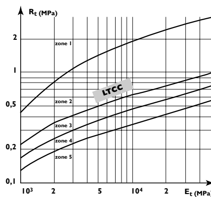
Figure 1 : Classes de résistance. E_t , R_t sont mesurés à 180 jours. (Extrait du Manuel de conception SETRA-LCPC .)
