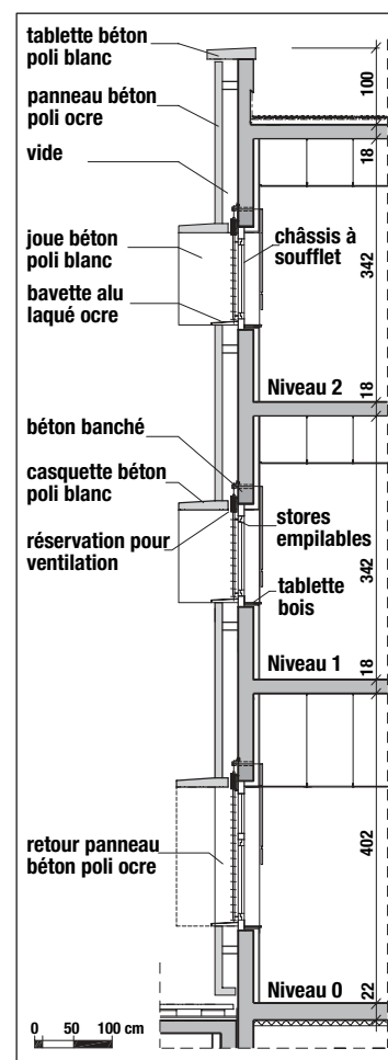
III Coupe de détail sur façade sud
